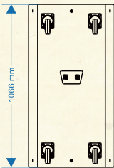
后视图
